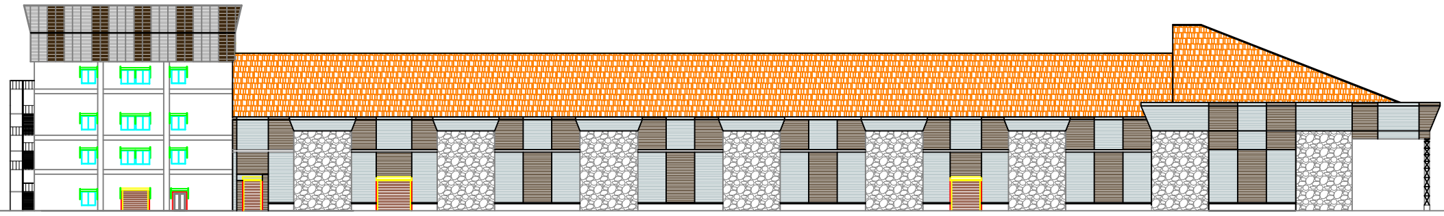
ELEVATION
